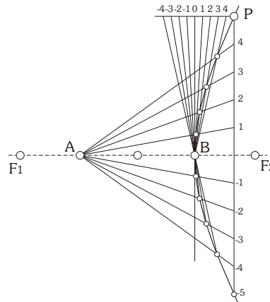
Por proxeccións, dados o Diámetro maior, os focos e un punto P
