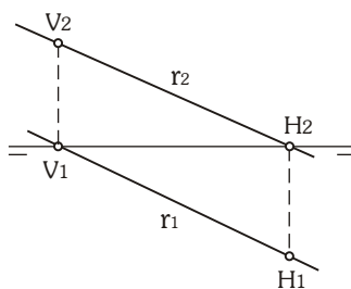
Puntos notabeis dunha recta: Trazas (puntos de cota=0 e de distancia=0) intersección da recta cos planos de proxección.
